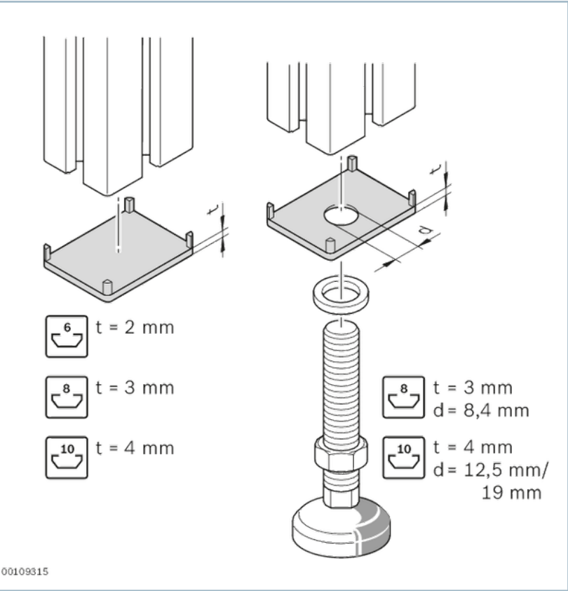
Einführung Strebenprofile
