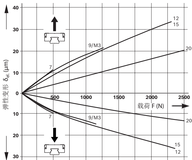
标准滚珠滑块 R0442
