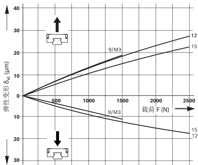
宽型滚珠滑块 R0443
