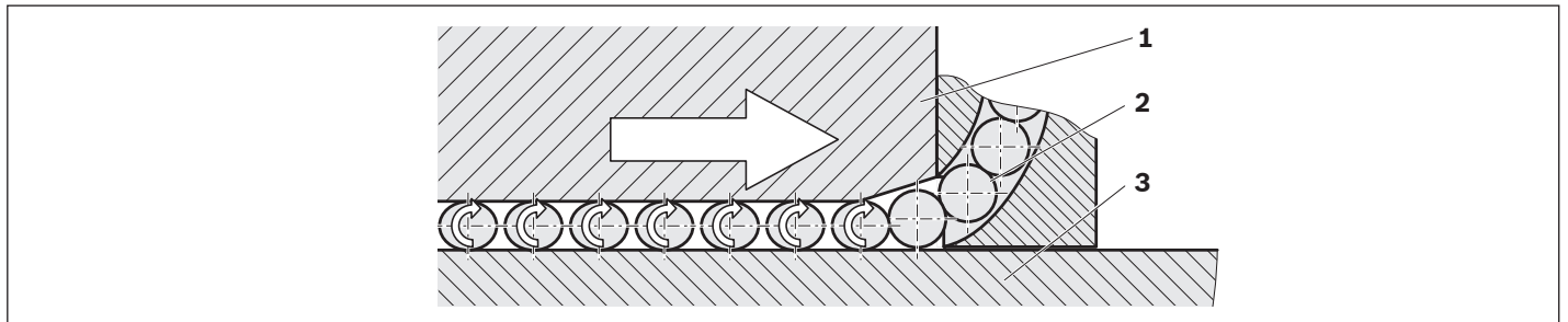
1) 滚珠滑块 2) 滚珠 3) 滚珠导轨
