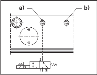
a) 空气接口 b) 空气滤清器 公称直径：最小 6 mm
