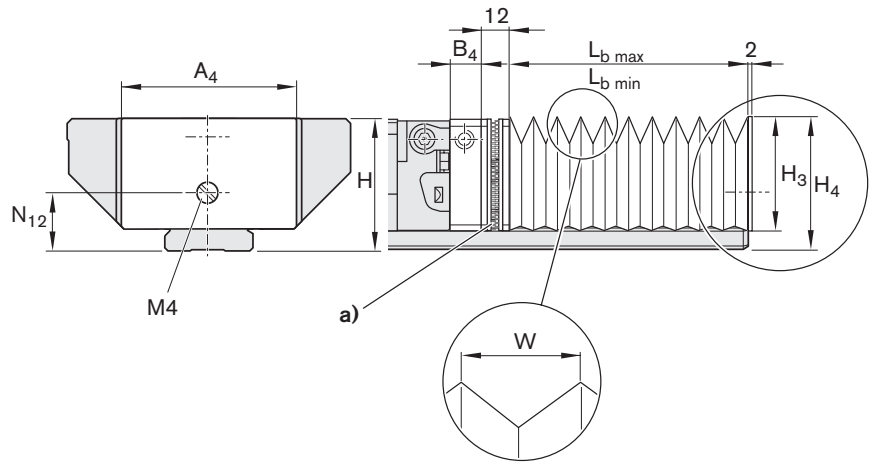
耐高温波纹罩 2) (请注意安装高度)
