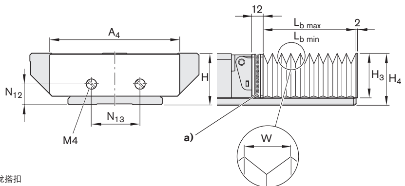
宽波纹罩
