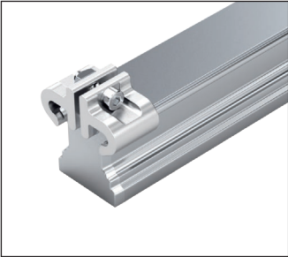
带防护带和铝制防护带扣的滚珠导轨
