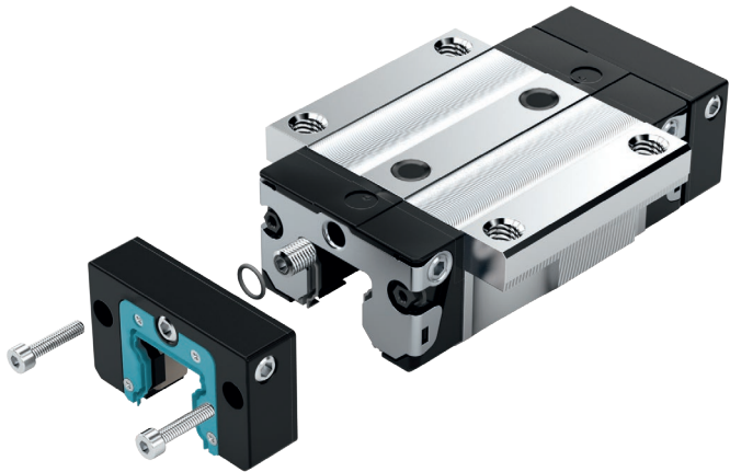
配有两个前置润滑单元的标准滚珠滑块
