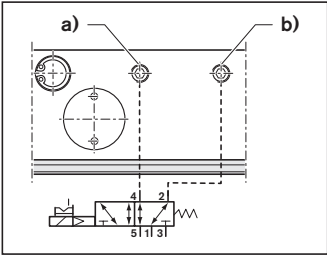
a) 空气接口 b) 附加空气接口 公称直径：最小 6 mm
