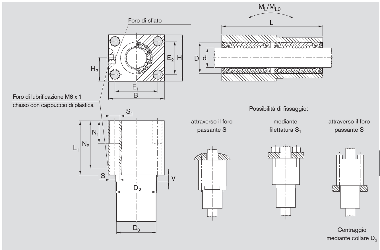
Dimensioni (mm)
