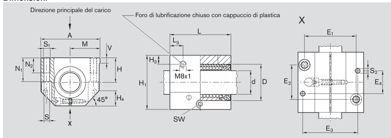
Dimensioni (mm)
