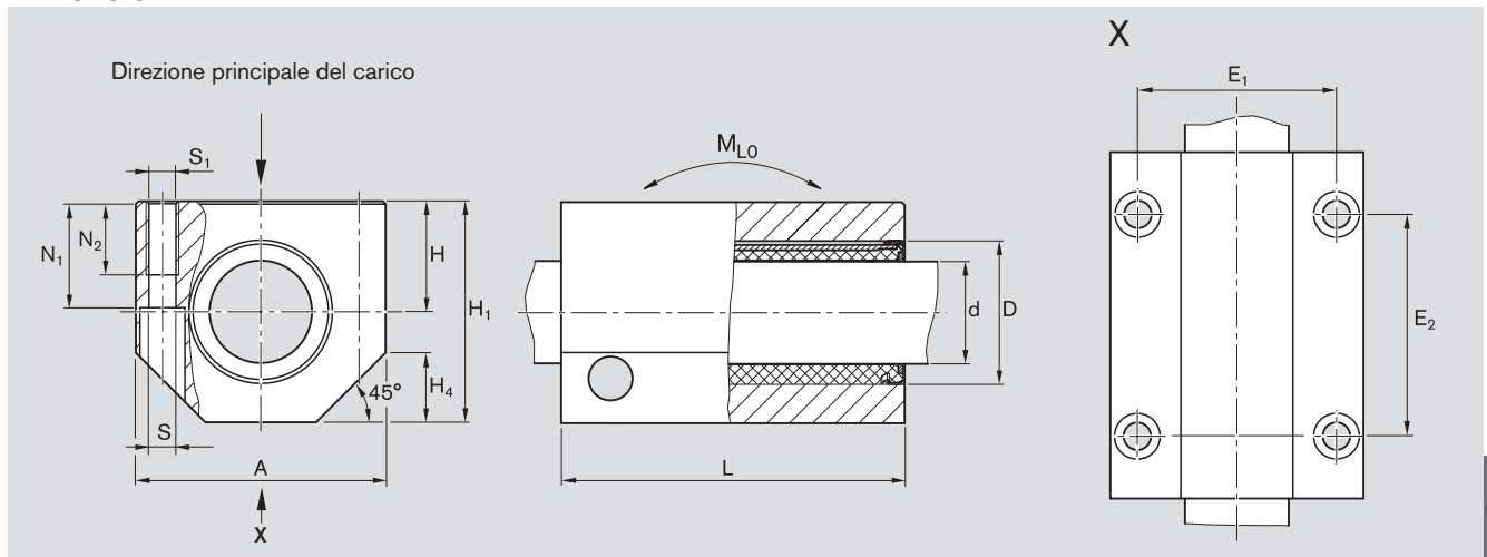
Dimensioni (mm)
